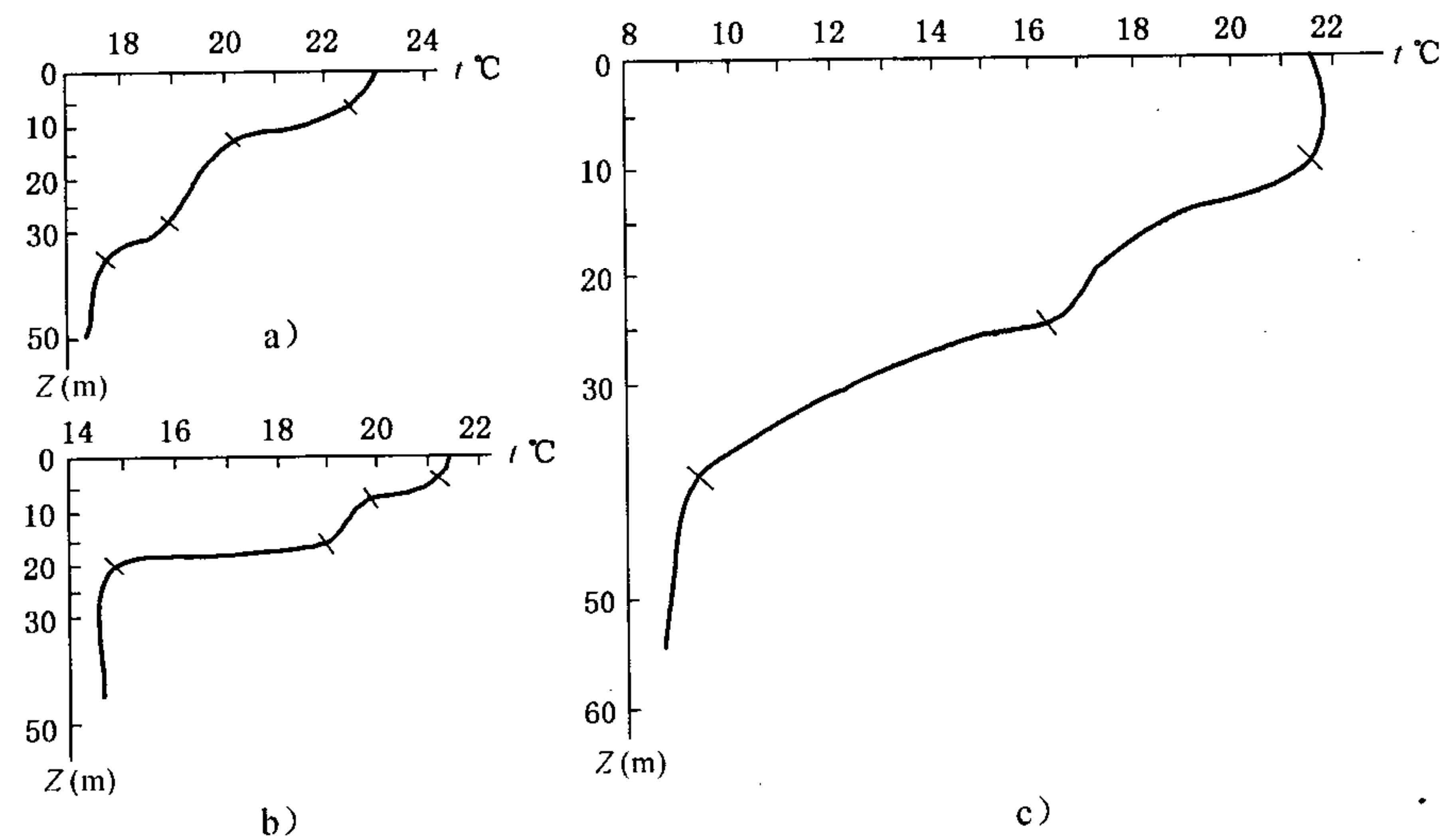
图 A.3 双跃层位置示意图
