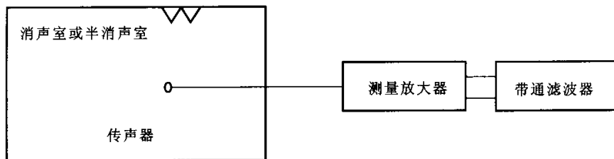
图 4 本底噪声测量装置方框图
