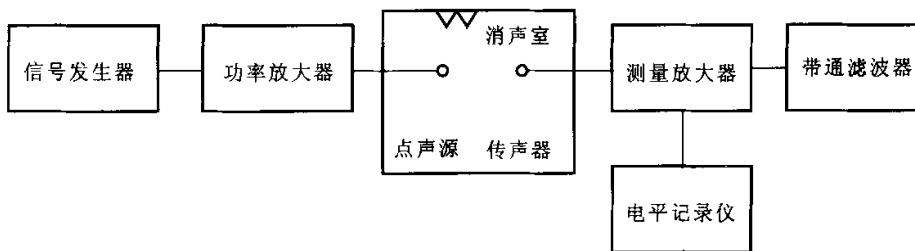
图 1 消声室自由声场频率范围和空间范围的测量装置方框图
