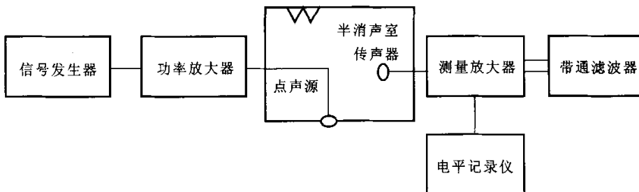
图 2 半消声室自由声场频率范围和空间范围的测量装置方框图
