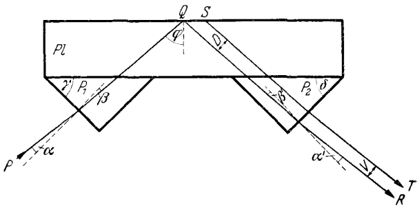
Abb. 7. Wirklicher Verlauf der Strahlen
