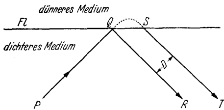
Abb. 1. Prinzip des Strahlenverlaufes
