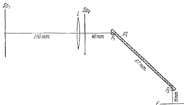
Abb. 6. Aufbau der Apparatur
