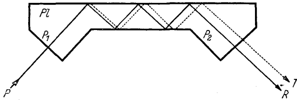
Abb. 4 Prinzip der Vielfachreflexion
